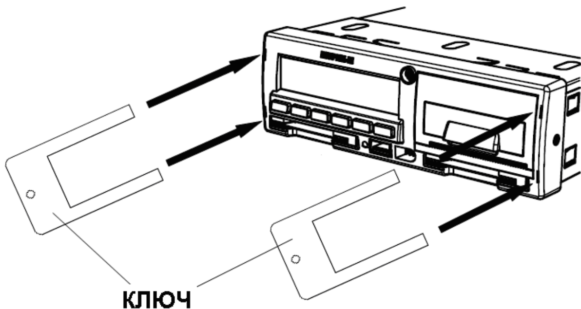
Рисунок 3 – Извлечение тахографа
